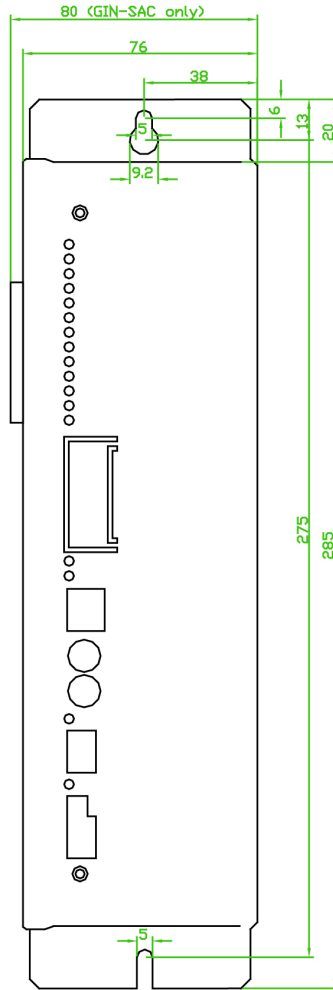
Fig. 3: SAC 5A
