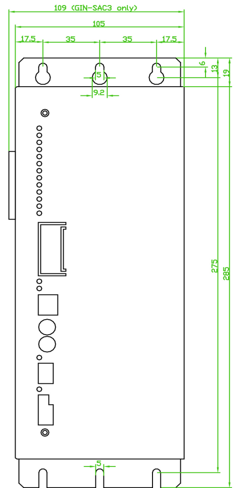
Fig. 4: SAC 16/24A
